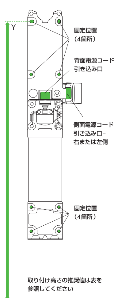
背面図
